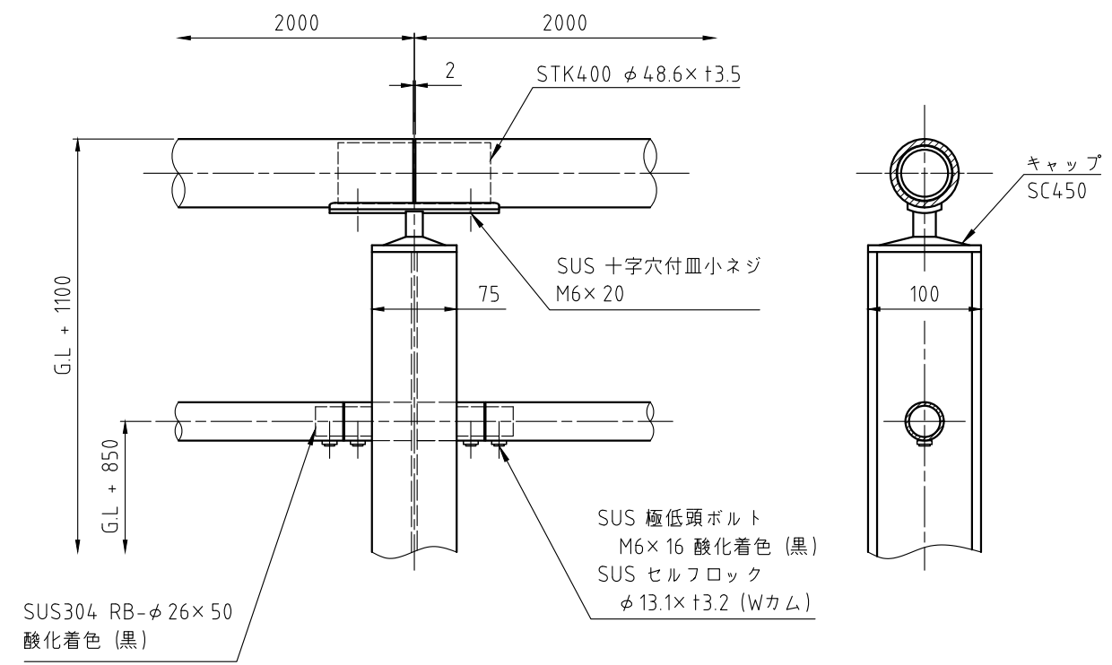
詳細図 S=1:6
