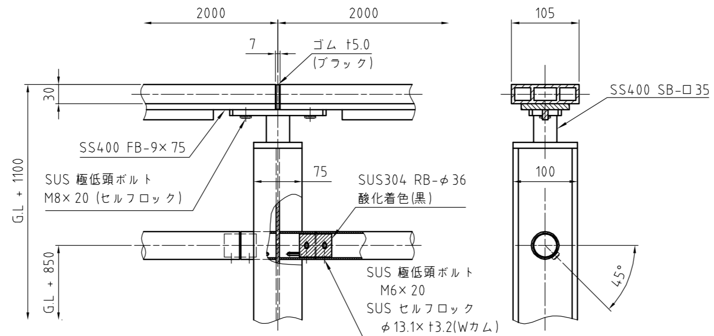
詳細図 S=1:6
