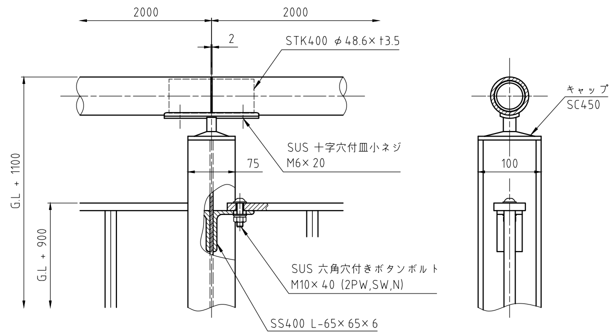
詳細図 S=1:6
