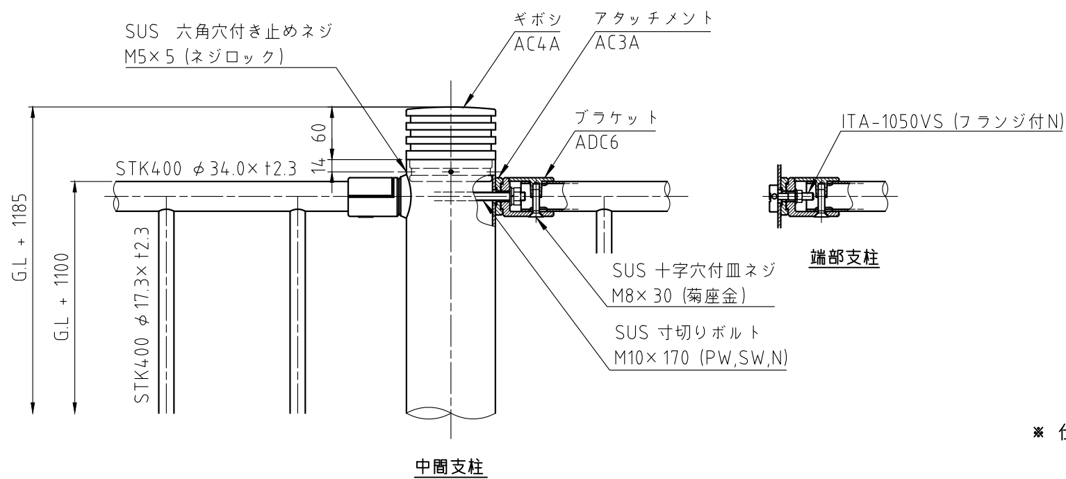
詳細図 S=1:6
