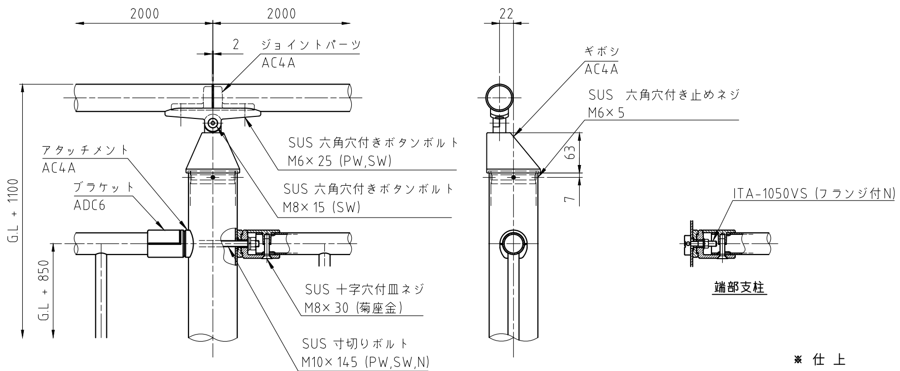
詳細図 S=1:6
