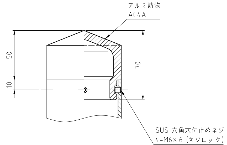
A-A'矢視図 支柱頂部詳細図 S=1:2
