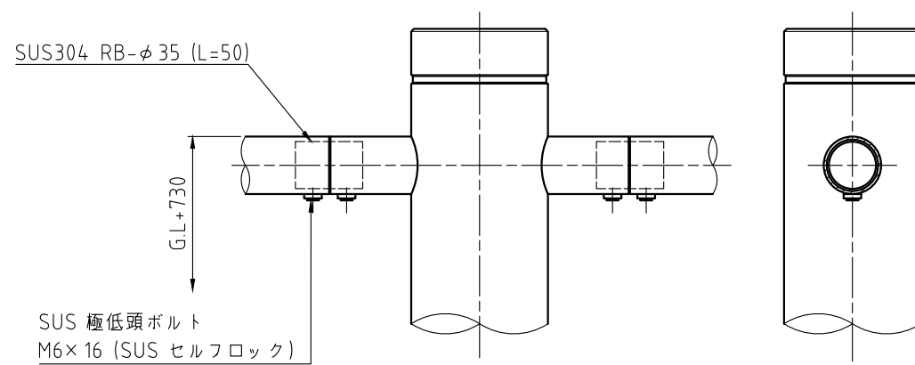
支柱頂部詳細図 S=1:5
