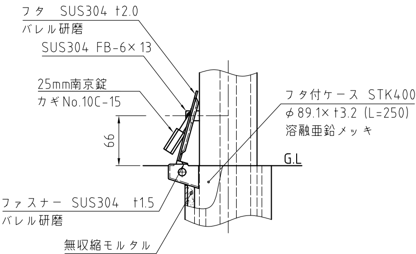
施錠部詳細図 S=1:5
