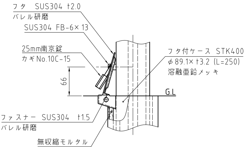
施錠部詳細図 S=1:5
