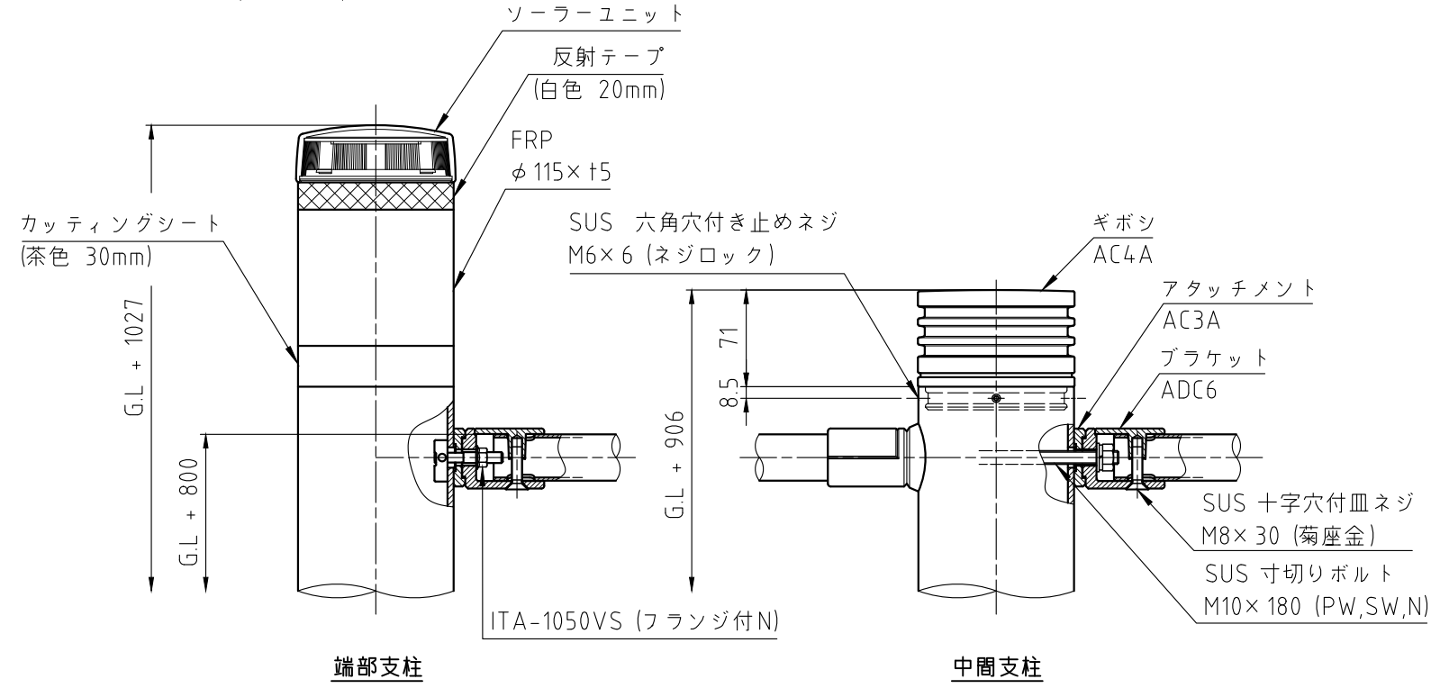
詳細図 S=1:5
