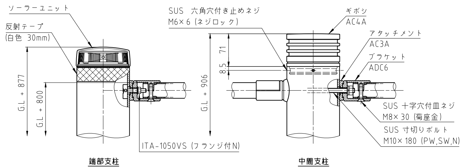
詳細図 S=1:5
