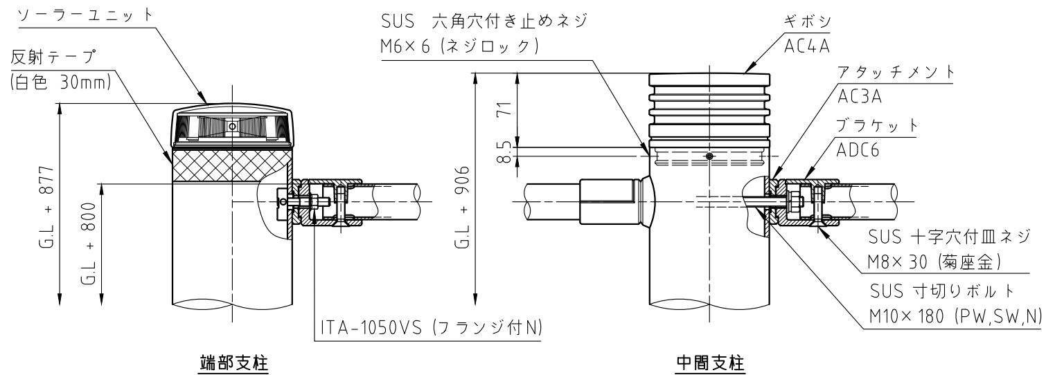
詳細図 S=1:5
