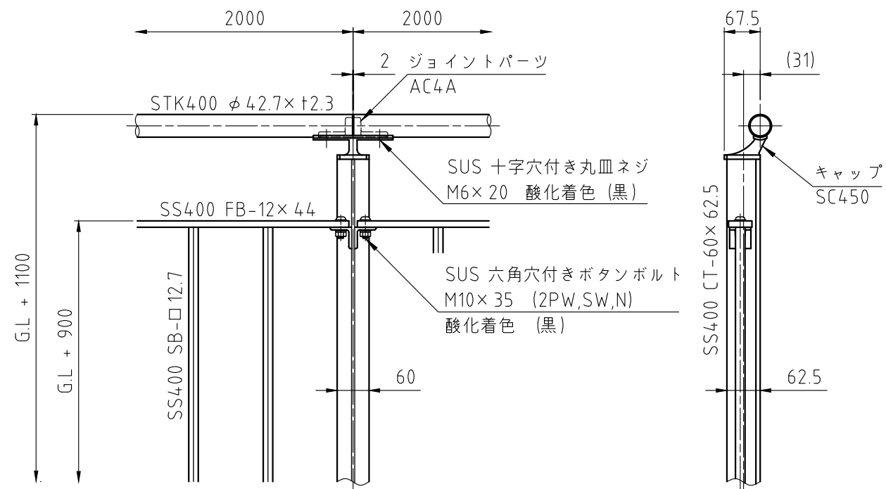
詳細図 S=1:10
