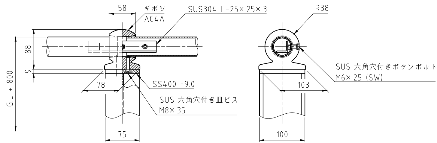
詳細図 S=1:5
