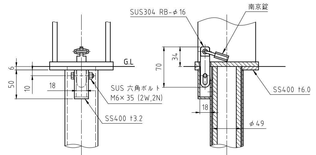
施錠部詳細図 S=1:4
